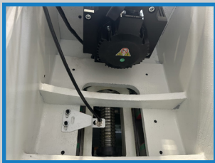
Une vis à billes centrale +servomoteur
