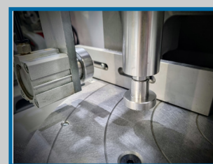
Vérin de bridage
