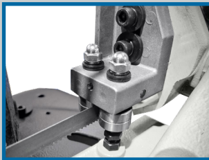
Guidage de la lame
