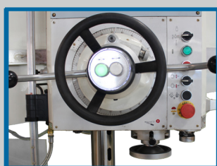
Commande de verrouillage des axes
