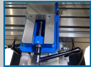
Étau de fraisage
